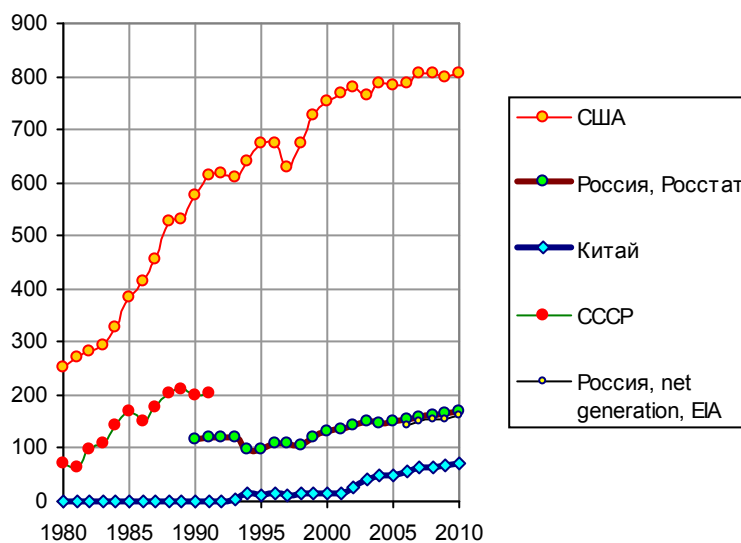
Производство электроэнергии на атомных электростанциях, млрд. кВт-час. Источник: Energy Information Administration, EIA
