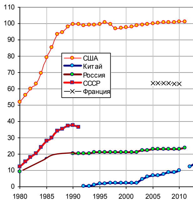
Установленная мощность атомных электростанций, млн. кВт. Источники: Росстат; Energy Information Administration, International Energy Annual.
