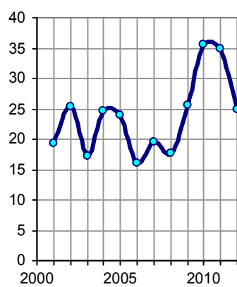
Ввод мощностей по переработке нефти в Китае (Newly Increased Production Capacity, Petroleum Extraction), млн. тонн. в год. Источник: National Bureau of Statistics of China.
