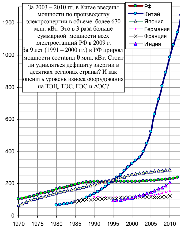
Мощность электростанций, млн. кВт. Источники: [1,4, 1,6]; National Bureau of Statistics of China; Japan Statistical Yearbook; Energy Information Administration (EIA).
