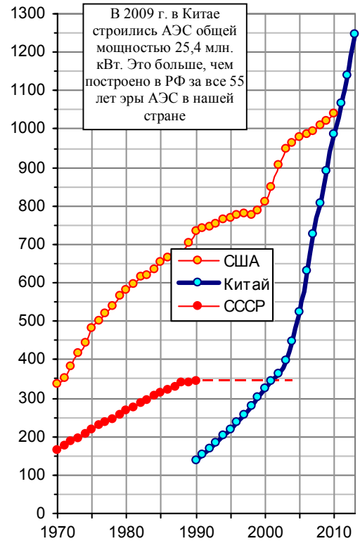
Установленная мощность электростанций в США, в Китае и в СССР, млн. кВт. Источники: U.S. Energy Information Administration (EIA), International Energy; U.S. Census Bureau, The 2011 Statistical Abstract; National Bureau of Statistics of China.
